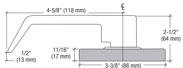
Passage Function (F 75)
