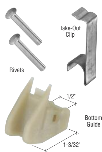
Bottom Guide
