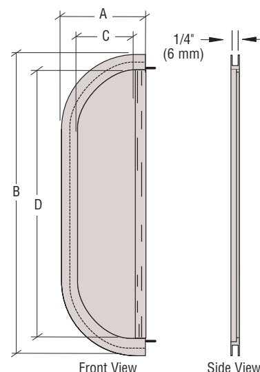
TP125 Template
