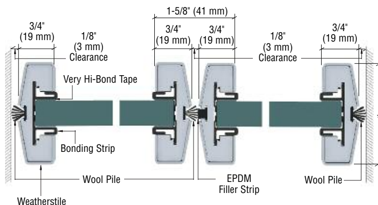
Double Door
