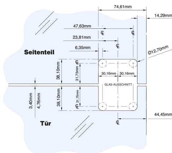
Ausschnitt Eckmontage, 3 - 5 mm Spaltmaß
