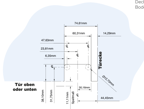
Ausschnitt Eckmontage, 11 mm Spaltmaß
