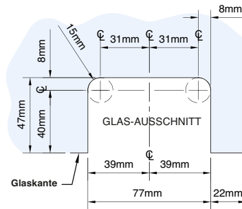
Ausschnitt Eckmontage
